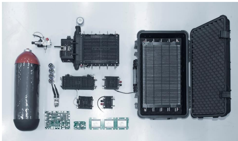
図2. Spectronik製 空冷式燃料電池Protiumシリーズと周辺機器
